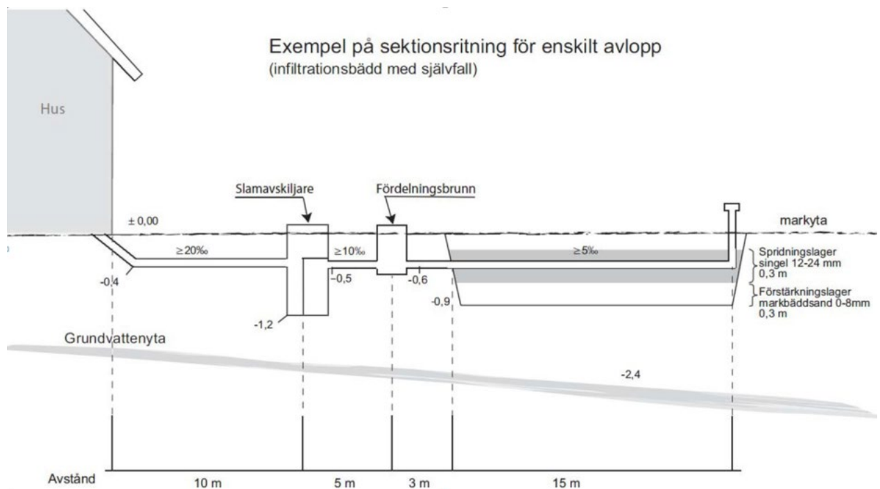
Bild: Exempel på hur en sektionsritning för en infiltrationsanläggning kan se ut. Skissen är ej skalendig.
